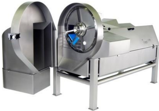
Lifis.2 Hochleistungsanlage
