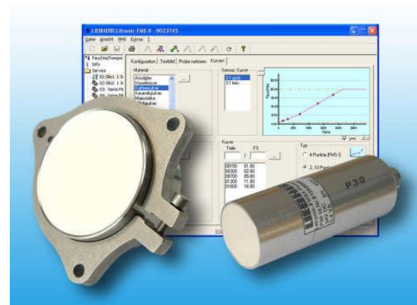
Litronic-FMS II bestehend aus intelligentem Sensor, Auswerteelektronik und Software.
